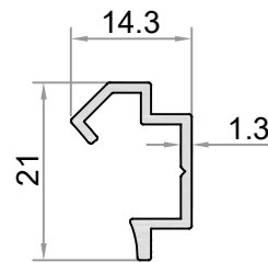
W-546 AĞIRLIK / WEIGHT (KG/M.) 0,152
