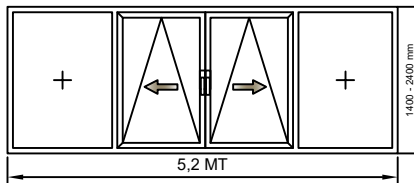
480498 (380498) ŞEMA C / 2,6 MT RAY
