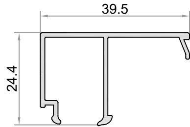
W-520-a AĞIRLIK / WEIGHT (KG/M.) 0,317
