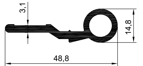
NO:7246 AĐIRLIK:583 gr/m
