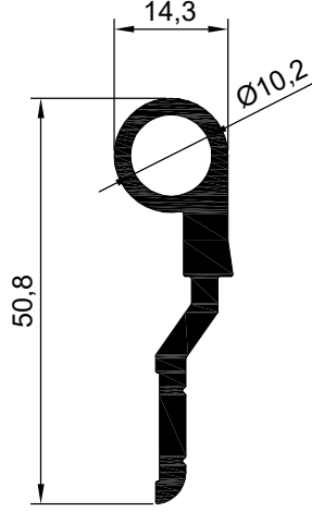
NO : 3373 AGIRLIK : 0.629 kg/m
