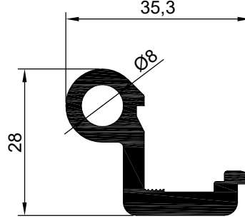
NO : 2106 AGIRLIK : 0.739 kg/m
