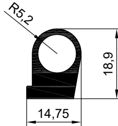
NO : 5345 AGIRLIK : 0.375 kg/m
