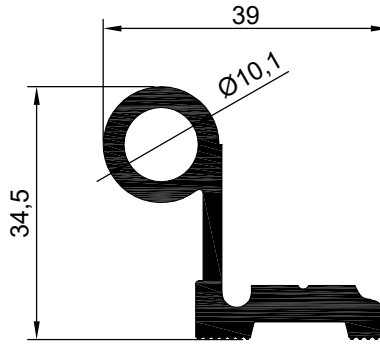
NO : 2095 AGIRLIK : 0.808 kg/m
