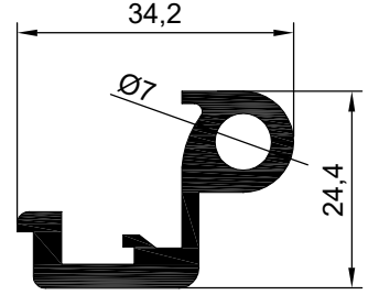
NO : 2063 AGIRLIK : 0.623 kg/m
