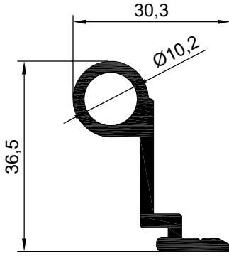
NO : 2094 AGIRLIK : 0.543 kg/m
