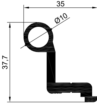
NO : 2105 AGIRLIK : 0.726 kg/m
