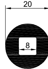
NO : 2289 AGIRLIK : 0.675 kg/m
