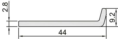
FP393 AĞIRLIK / WEIGHT (KG/M.) 0,368
