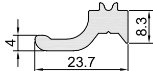
FP378 AĞIRLIK / WEIGHT (KG/M.) 0,318
