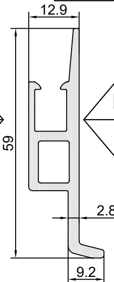
FP392 AĞIRLIK / WEIGHT (KG/M.) 0,338
