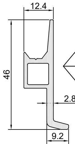
FP391 AĞIRLIK / WEIGHT (KG/M.) 0,308
