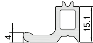
FP380 AĞIRLIK / WEIGHT (KG/M.) 0,354
