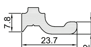
FP383 AĞIRLIK / WEIGHT (KG/M.) 0,343
