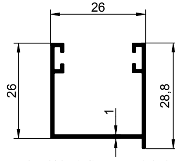
NO : 644 AGIRLIK : 0.259 kg/m
