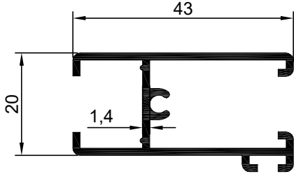
NO : 1358 AGIRLIK : 0.508 kg/m
