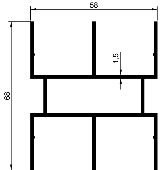
NO : 1356 AGIRLIK : 1.195 kg/m
