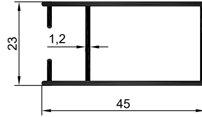
NO : 1888 AGIRLIK : 0.462 kg/m
