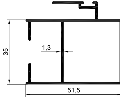
NO : 1883 AGIRLIK : 0.788 kg/m
