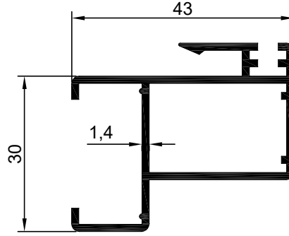
NO : 1363 AGIRLIK : 0.637 kg/m
