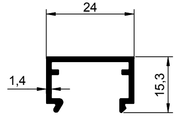
NO : 1457 AGIRLIK : 0.232 kg/m
