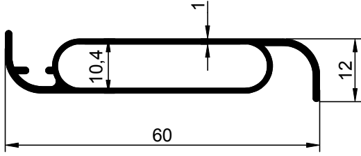
NO : 1885 AGIRLIK : 0.402 kg/m
