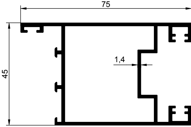
NO : 1447 AGIRLIK : 1.129 kg/m
