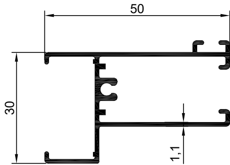
NO : 1621 AGIRLIK : 0.511 kg/m
