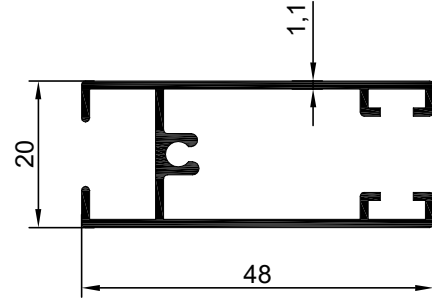
NO : 1884 AGIRLIK : 0.464 kg/m
