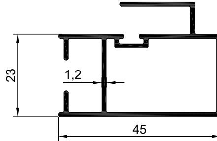
NO : 1889 AGIRLIK : 0.589 kg/m
