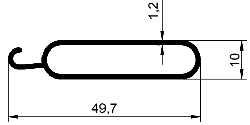
NO : 957 AGIRLIK : 0.333 kg/m
