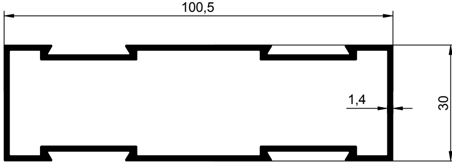
NO : 1446 AGIRLIK : 1.096 kg/m
