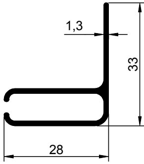
NO : 1057 AGIRLIK : 0.312 kg/m
