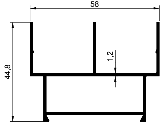
NO : 2552 AGIRLIK : 0.718 kg/m
