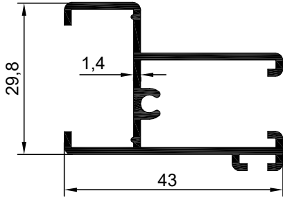
NO : 1359 AGIRLIK : 0.544 kg/m
