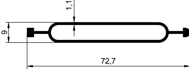
NO : 1128 AGIRLIK : 0.437 kg/m
