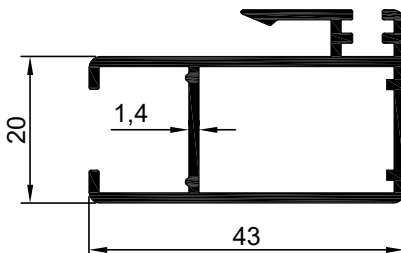
NO : 1362 AGIRLIK : 0.603 kg/m
