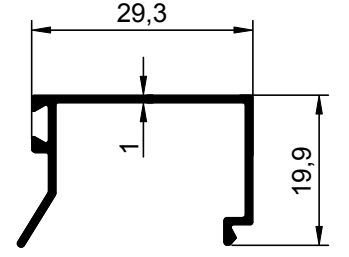
NO : 599 AGIRLIK : 0.209 kg/m
