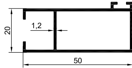
NO : 1615 AGIRLIK : 0.494 kg/m
