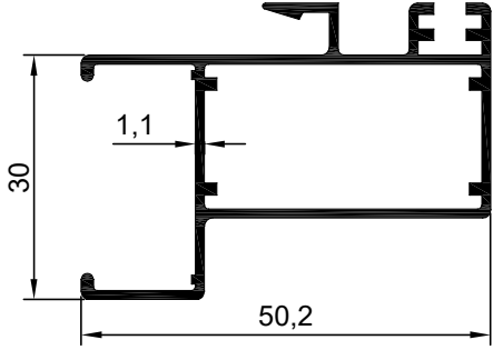
NO : 1618 AGIRLIK : 0.589 kg/m
