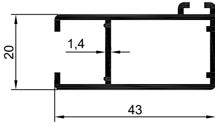
NO : 1360 AGIRLIK : 0.516 kg/m
