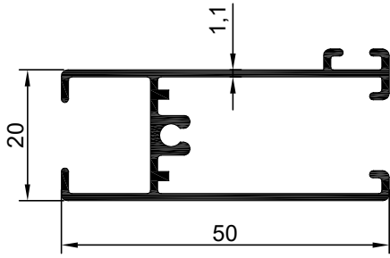
NO : 1620 AGIRLIK : 0.489 kg/m
