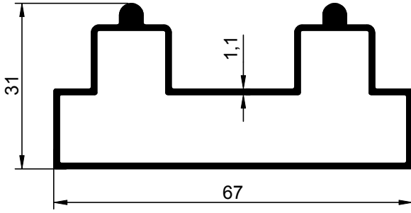
NO : 2511 AGIRLIK : 0.697 kg/m
