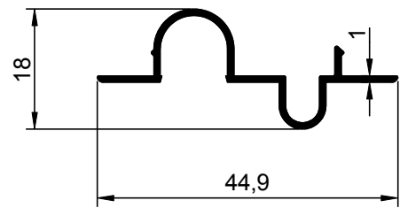
NO : 1666 AGIRLIK : 0.205 kg/m
