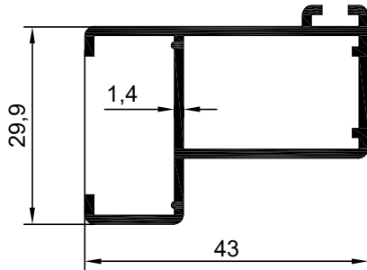
NO : 1361 AGIRLIK : 0.553 kg/m
