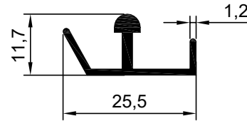
NO : 1616 AGIRLIK : 0.193 kg/m
