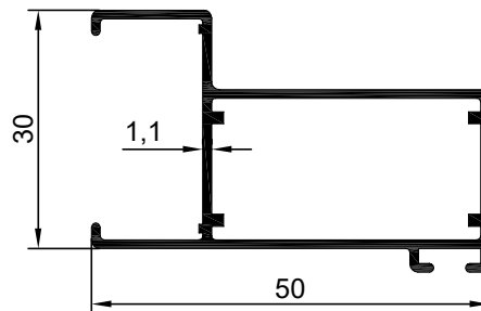
NO : 1617 AGIRLIK : 0.497kg/m
