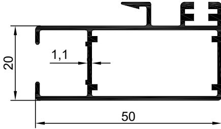
NO : 1619 AGIRLIK : 0.575 kg/m
