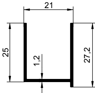
NO : 948 AGIRLIK : 0.229 kg/m
