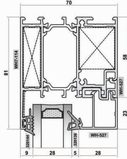
ALTERNATİF EŞİK DETAYI: 3 ALTERNATIVE SILL DETAIL NO: 3
