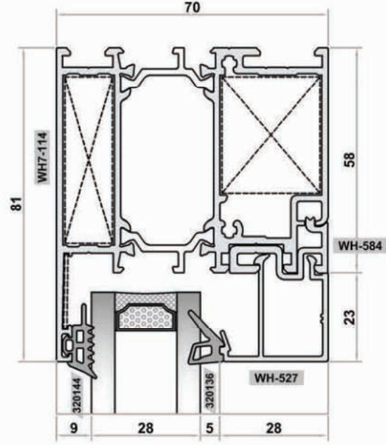
ALTERNATİF EŞİK DETAYI: 2 ALTERNATIVE SILL DETAIL NO: 2
