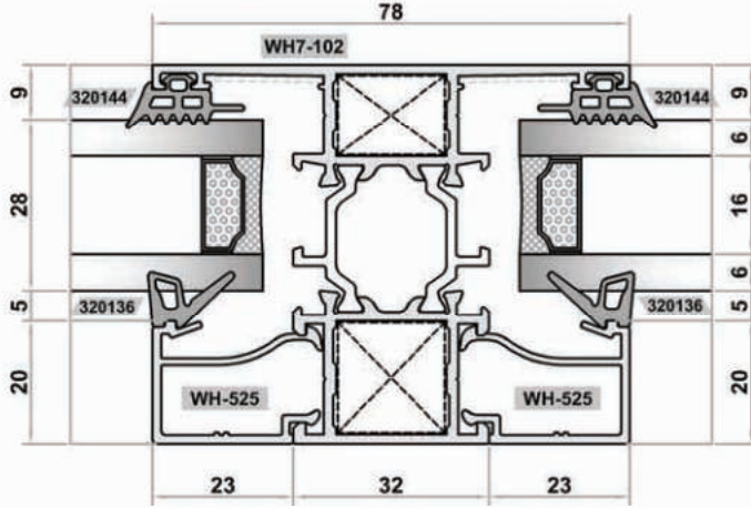
ALTERNATİF ORTA KAYIT DETAYI: 1 ALTERNATIVE TRANSOM DETAIL NO: 1
