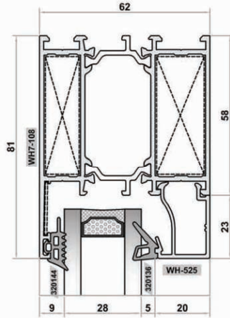
ALTERNATİF EŞİK DETAYI: 3 ALTERNATIVE SILL DETAIL NO: 3
