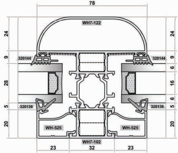
ALTERNATİF ORTA KAYIT DETAYI: 2 ALTERNATIVE TRANSOM DETAIL NO: 2
