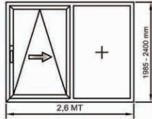
480483 (380483) ŞEMA A / SOL / 2,6 MT RAY
