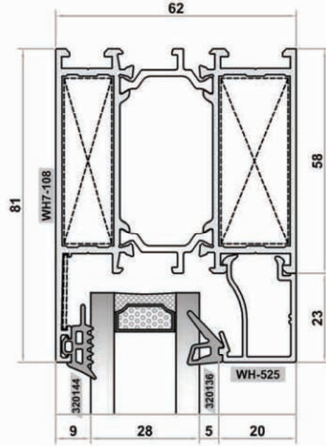
ALTERNATİF EŞİK DETAYI: 2 ALTERNATIVE SILL DETAIL NO: 2
