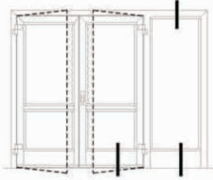
ALTERNATİF EŞİK DETAYI: 2 ALTERNATIVE SILL DETAIL NO: 2
