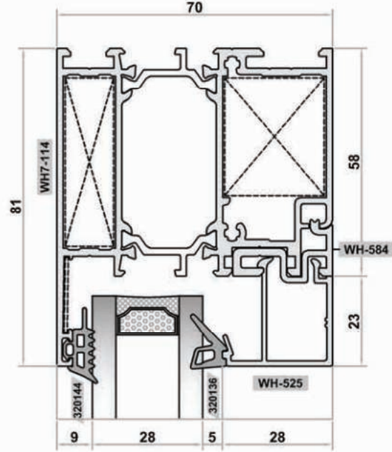
ALTERNATİF EŞİK DETAYI: 3 ALTERNATIVE SILL DETAIL NO: 3
