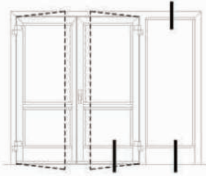
ALTERNATİF EŞİK DETAYI: 3 ALTERNATIVE SILL DETAIL NO: 3
