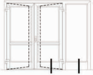
ALTERNATİF EŞİK DETAYI: 3 ALTERNATIVE SILL DETAIL NO: 3
