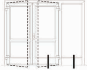
ALTERNATİF EŞİK DETAYI: 2 ALTERNATIVE SILL DETAIL NO: 2
