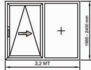
480484 (380484) ŞEMA A / SOL / 3,2 MT RAY
