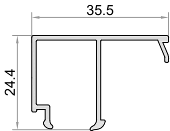
W-519-a AĞIRLIK / WEIGHT (KG/M.) 0,304
