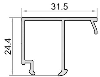
W-518-a AĞIRLIK / WEIGHT (KG/M.) 0,291
