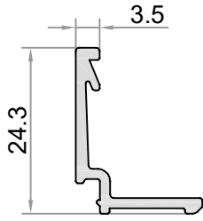
W-511-a AĞIRLIK / WEIGHT (KG/M.) 0,203
