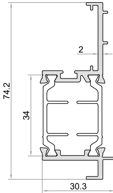
W8-506 AĞIRLIK / WEIGHT (KG/M.) 0,940 (PVC) 0,918 (POL.)
