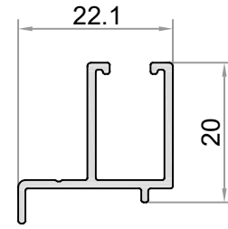
W-543 AĞIRLIK / WEIGHT (KG/M.) 0,213
