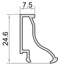
W-512-a AĞIRLIK / WEIGHT (KG/M.) 0,211
