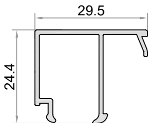
W-522-a AĞIRLIK / WEIGHT (KG/M.) 0,284
