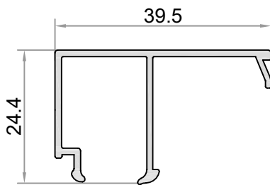
W-520-a AĞIRLIK / WEIGHT (KG/M.) 0,317
