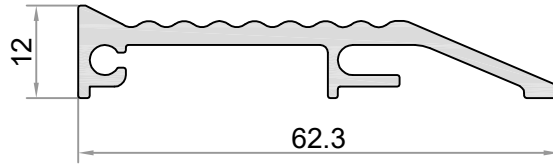
W-545 AĞIRLIK / WEIGHT (KG/M.) 0,578
