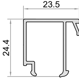
W-516-a AĞIRLIK / WEIGHT (KG/M.) 0,265
