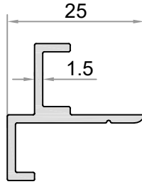
W-538 AĞIRLIK / WEIGHT (KG/M.) 0,249
