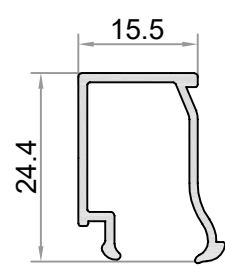
W-514-a AĞIRLIK / WEIGHT (KG/M.) 0,225
