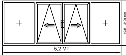
480489 (380489) ŞEMA C / 2,6 MT RAY
