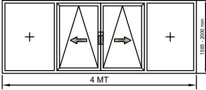
480485 (380485) ŞEMA C / 2 MT RAY
