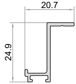
W-558 AĞIRLIK / WEIGHT (KG/M.) 0,173
