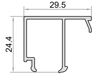
W-522-a AĞIRLIK / WEIGHT (KG/M.) 0,284
