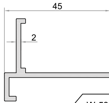
W-536 AĞIRLIK / WEIGHT (KG/M.) 0,292
