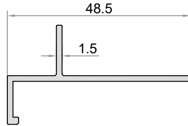
W-542 AĞIRLIK / WEIGHT (KG/M.) 0,306
