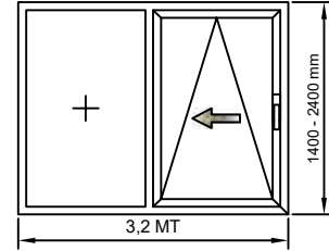
480493 (380493) ŞEMA A / SAĞ / 3,2 MT RAY
