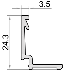
W-511-a AĞIRLIK / WEIGHT (KG/M.) 0,203
