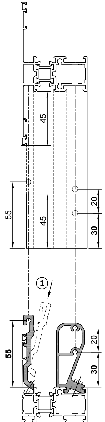
W-617 (1,154 kg/m.)
