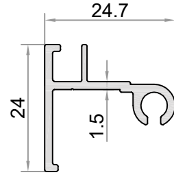
W3-509 AĞIRLIK / WEIGHT (KG/M.) 0,271
