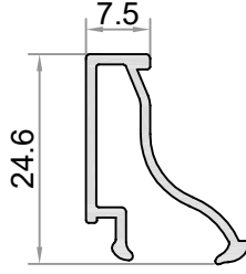
W-512-a AĞIRLIK / WEIGHT (KG/M.) 0,211
