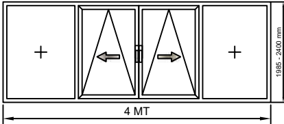
480488 (380488) ŞEMA C / 2 MT RAY
