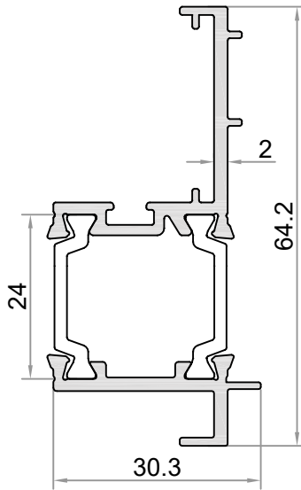
W6-506 AĞIRLIK / WEIGHT (KG/M.) 0,843 (PVC) 0,829 (POL.)
