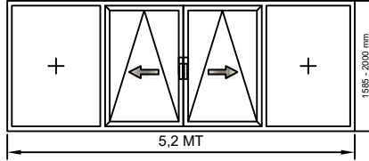
480486 (380486) ŞEMA C / 2,6 MT RAY
