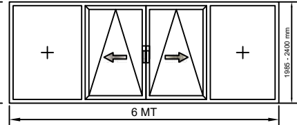
480490 (380490) ŞEMA C / 3,2 MT RAY
