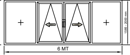
480487 (380487) ŞEMA C / 3,2 MT RAY
