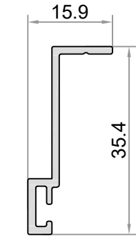
W-559 AĞIRLIK / WEIGHT (KG/M.) 0,216
