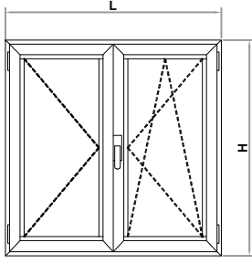
ÇİFT KANATLI ÇİFT AÇILIM PENCERE DOUBLE SASH TILT&TURN OPENING WINDOW
