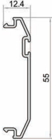
W-505 AĞIRLIK / WEIGHT (KG/M.) 0,271
