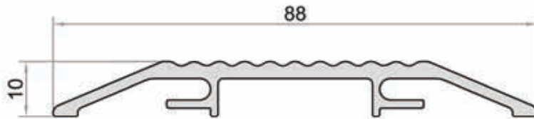
W-544 AĞIRLIK / WEIGHT (KG/M.) 0,728
