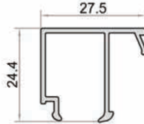
W-517-a AĞIRLIK / WEIGHT (KG/M.) 0,278
