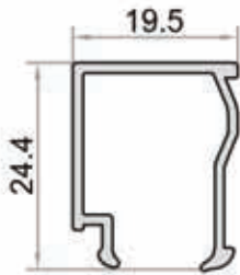
W-515-a AĞIRLIK / WEIGHT (KG/M.) 0,238
