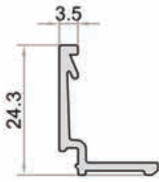
W-511-a AĞIRLIK / WEIGHT (KG/M.) 0,203
