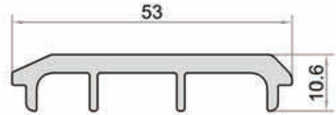
W-547 AĞIRLIK / WEIGHT (KG/M.) 0,621
