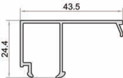
W-521-a AĞIRLIK / WEIGHT (KG/M.) 0,330
