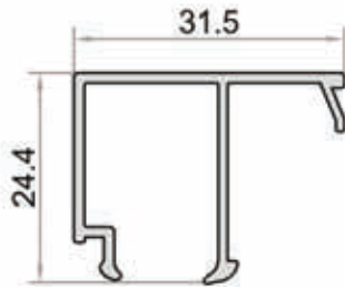
W-518-a AĞIRLIK / WEIGHT (KG/M.) 0,291
