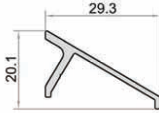
W-503 AĞIRLIK / WEIGHT (KG/M.) 0,211
