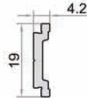
W1-508 AĞIRLIK / WEIGHT (KG/M.) 0,134
