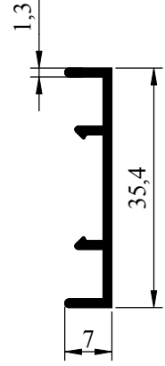
NO : 1690 AGIRLIK : 0.193 kg/m
