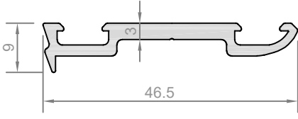
Profil No: SK78-304 Ağırlık : 383 gr/m
