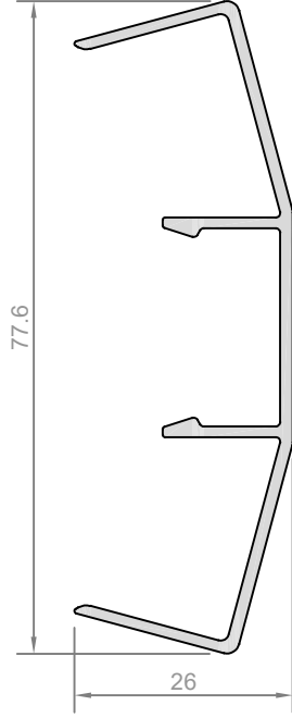
Profil No: KC0327 Ağırlık : 562 gr/m
