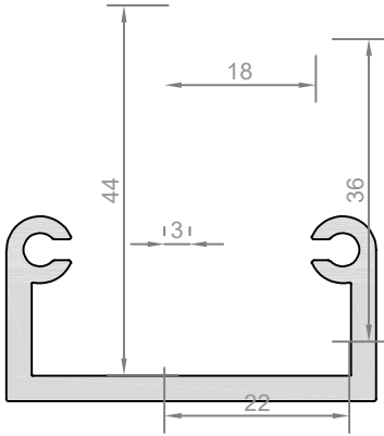
Profil No: SK50-301 Ağırlık : 731 gr/m
