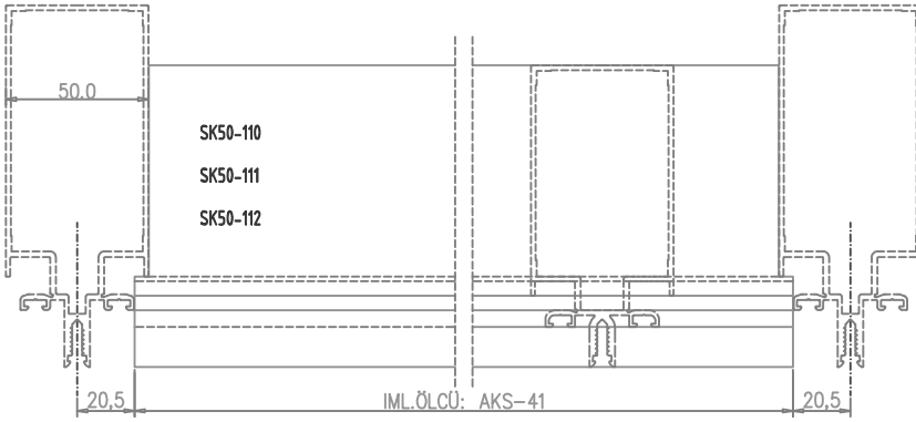
YATAY BASKI - KAPAK İMALAT BOYU
