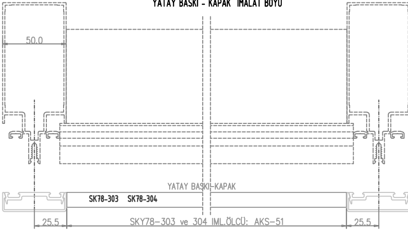
YATAY BASKI - KAPAK İMALAT BOYU
