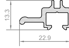
Profil No: EC0301 Ağırlık : 223 gr/m
