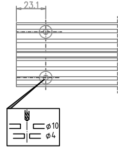
YATAY TASIYICI PROFİL KERTME ve DELİK DELME İŞLEMİ
