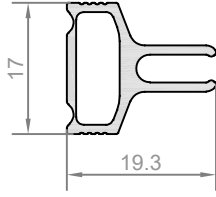
Profil No: EC0201 Ağırlık : 220 gr/m
