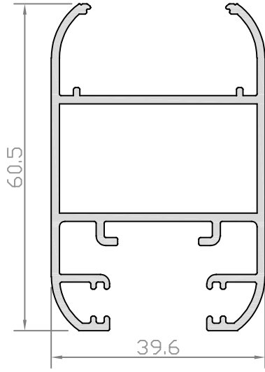
Profil No: S4-201 Ağırlık : 1016 gr/m lx : 8,84 cm 4 ly : 10,73 cm 4
