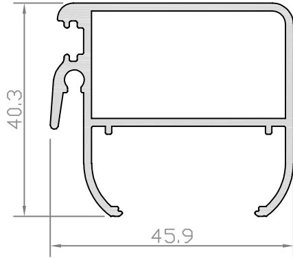
Profil No: S4-203 Ağırlık : 785 gr/m lx : 7,80 cm 4 ly : 4,08 cm 4
