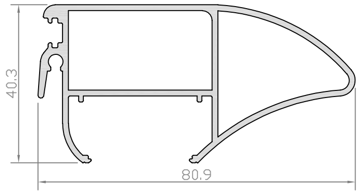
Profil No: S4-204 Ağırlık : 1119 gr/m lx : 24,00 cm 4 ly : 5,53 cm 4
