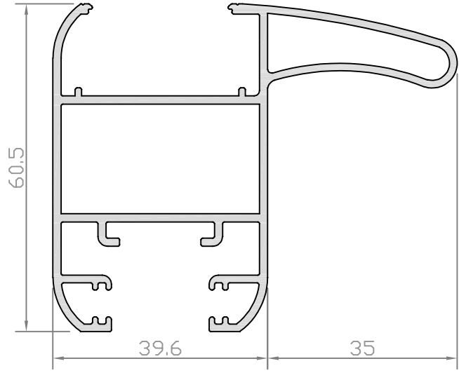
Profil No: S4-202 Ağırlık : 1314 gr/m lx : 21,76 cm 4 ly : 16,31 cm 4
