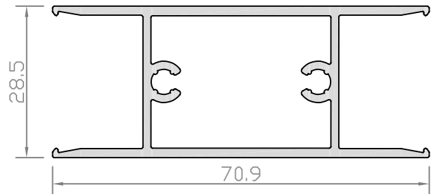
Profil No: S4-206 Ağırlık : 962 gr/m lx : 4,76 cm 4 ly : 12,57 cm 4
