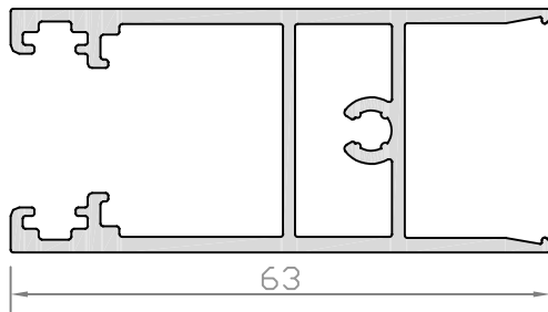
Profil No: S4-205 Ağırlık : 959 gr/m lx : 4,80 cm 4 ly : 10,50 cm 4
