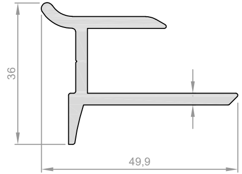
Profil No: OB1-203 ⚠ Ağırlık : 798 gr/m ⚠ İşaretti profil için satış temsilcinizden bilgi alınız.
