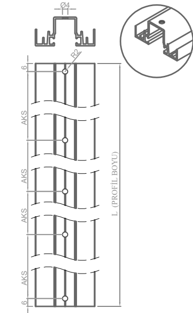
1-AHŞAP PANEL SAĞ SOL YAN PROFİLİ
