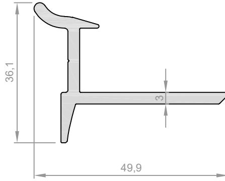
Profil No: OB1-202 Ağırlık : 666 gr/m
