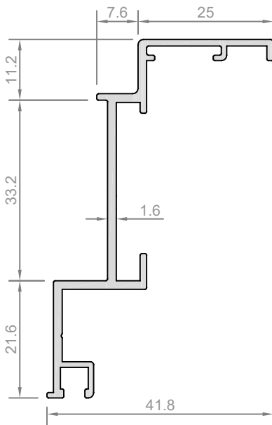
Profil No: MNF-104 Ağırlık : 540 gr/m
