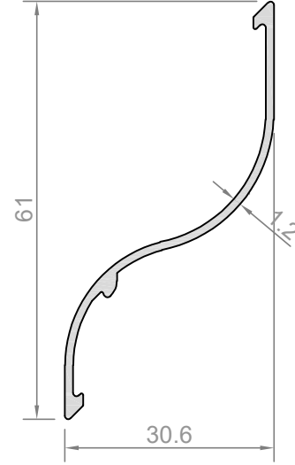
Profil No: MNF-207 Ağırlık : 277 gr/m
