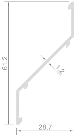
Profil No: MNF-208 Ağırlık : 275 gr/m
