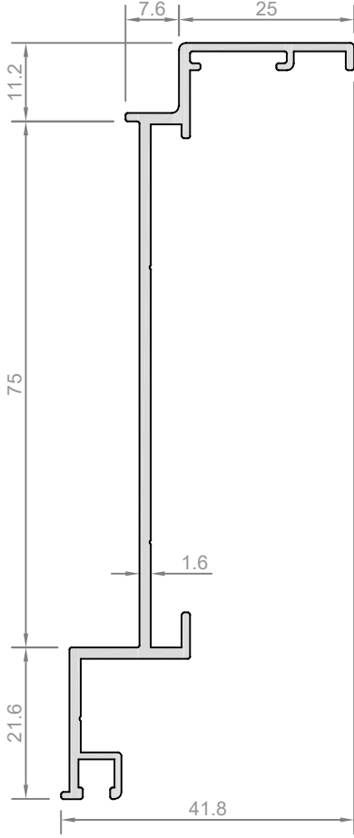
Profil No: MNF-101 Ağırlık : 721 gr/m
