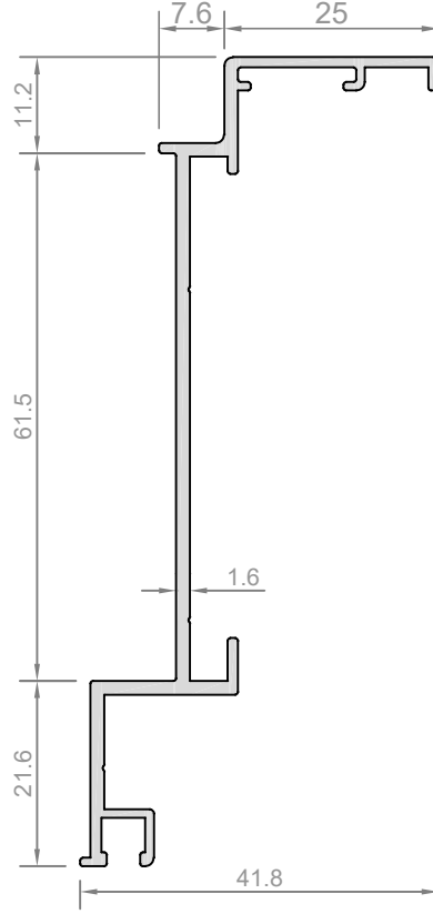
Profil No: MNF-102 Ağırlık : 663 gr/m
