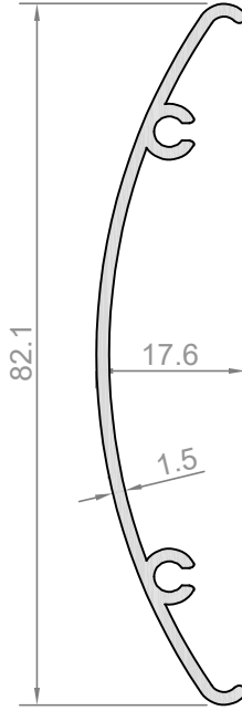
Profil No: MNF-206 Ağırlık : 460 gr/m
