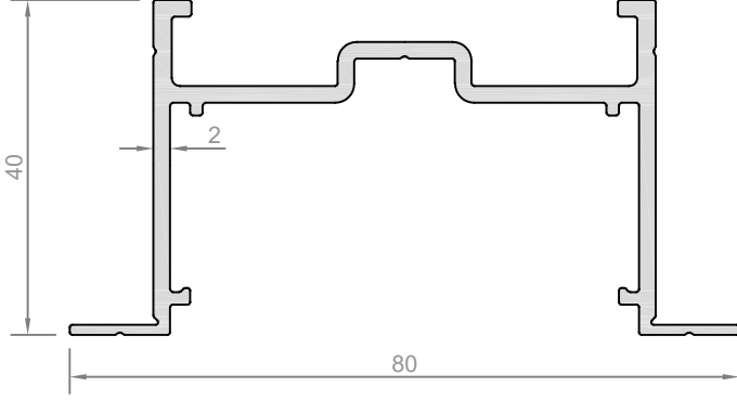
Profil No: KP0101 Ağırlık : 914 gr/m
