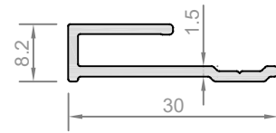
Profil No: KP0205 Ağırlık : 201 gr/m
