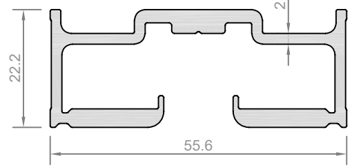
Profil No: KP0201 Ağırlık : 998 gr/m
