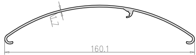
Profil No: GK-228 Ağırlık: 929gr/m
