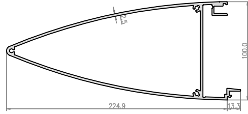
Profil No: GK-209 Ağırlık: 3868 gr/m
