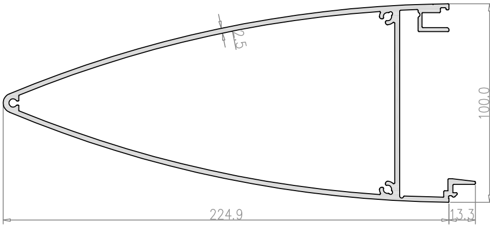
Profil No: GK-209 Ağırlık: 4271 gr/m
