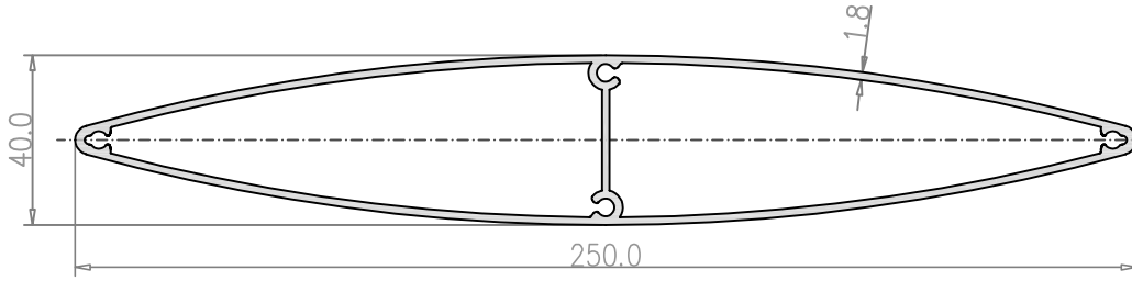
Profil No: GK-207 Ağırlık: 2784 gr/m
