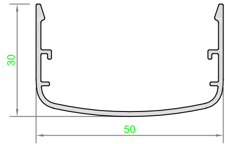
Profil No: KC0315 Ağırlık : 397 gr/m
