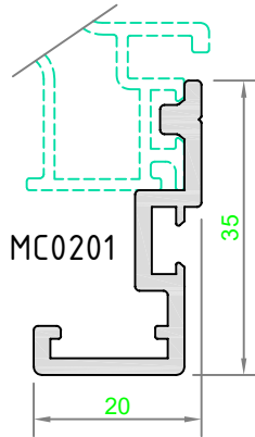
Profil No: MC0201 Ağırlık : 397 gr/m
