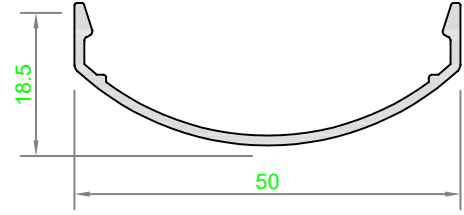
Profil No: KC0322 Ağırlık : 262 gr/m
