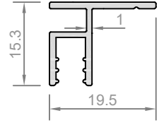
Profil No: COT-303 Ağırlık : 157 gr/m
