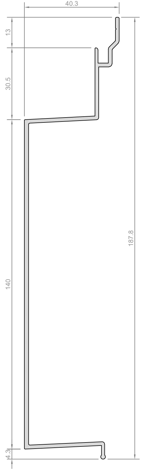
Profil No: COT-212 Ağırlık : 1206 gr/m
