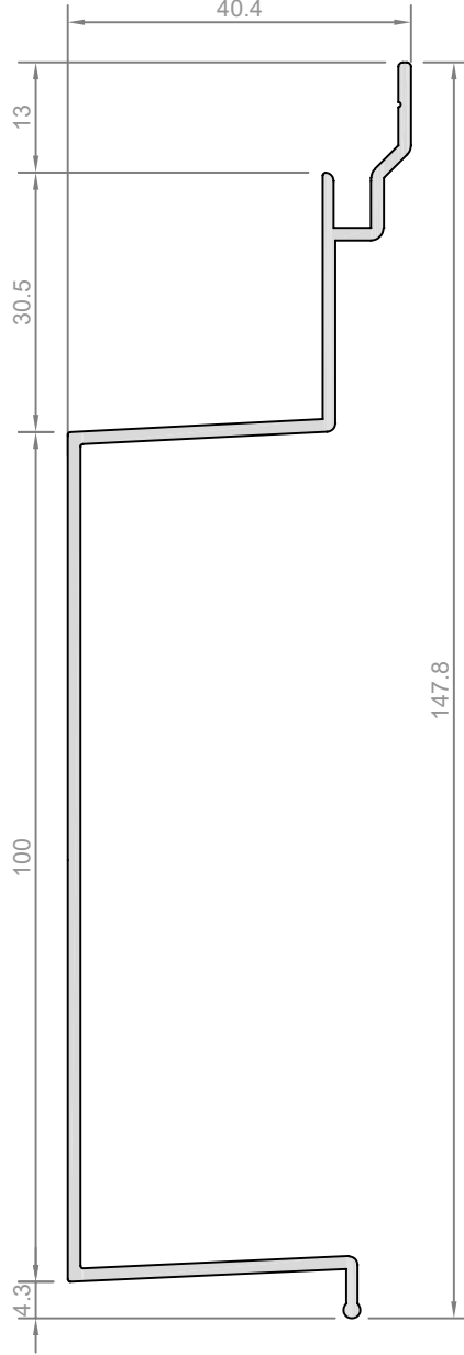
Profil No: COT-211 Ağırlık : 902 gr/m
