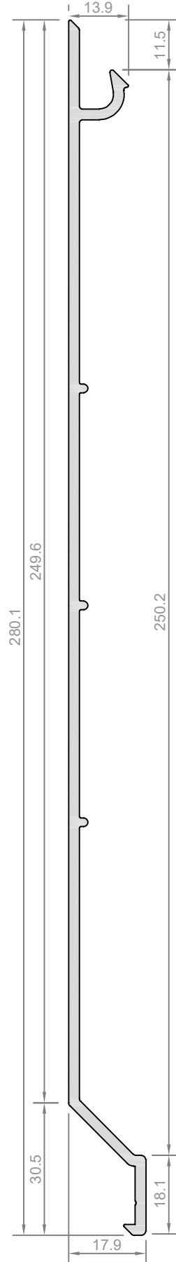
Profil No: COT-213 Ağırlık : 1572 gr/m
