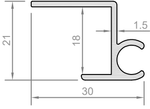
Profil No: COT-301 Ağırlık : 275 gr/m
