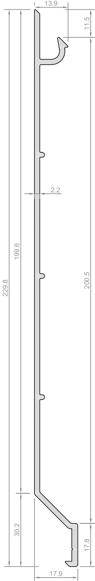
Profil No: COT-213 Ağırlık : 1572 gr/m
