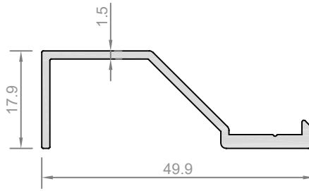
Profil No: COT-305 Ağırlık : 356 gr/m
