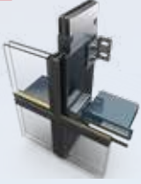
F50 Energy Yüksek Yalıtımlı Silikon Giydirmeye Cephe Sistemi
