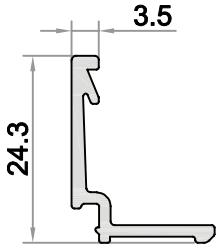
W-511-a AĞIRLIK / WEIGHT (KG/M.) 0,203
