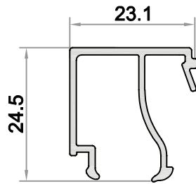
W-516 AĞIRLIK / WEIGHT (KG/M.) 0,278
