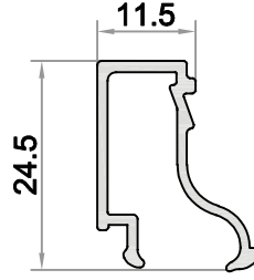
W-513 AĞIRLIK / WEIGHT (KG/M.) 0,229
