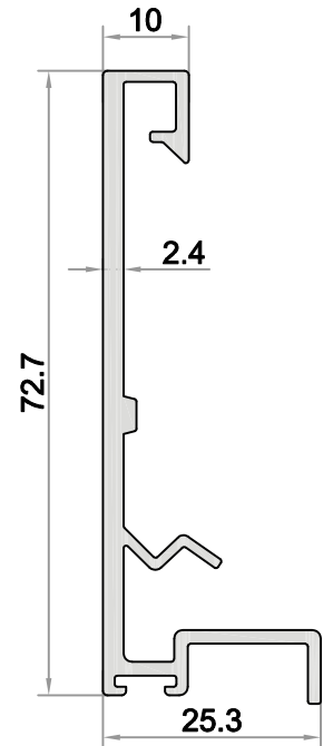
S3-517 AĞIRLIK / WEIGHT (KG/M.) 0,765
