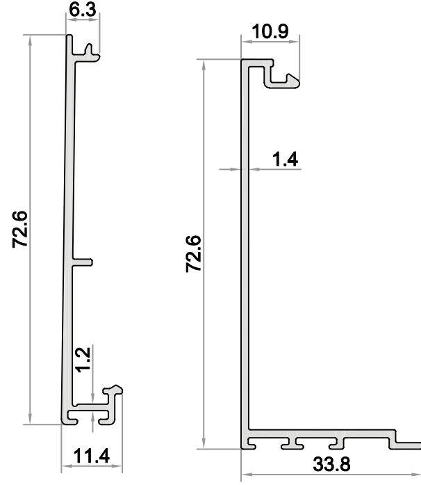
S3-512 AĞIRLIK / WEIGHT (KG/M.) 0,426
