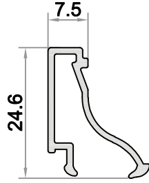
W-512 AĞIRLIK / WEIGHT (KG/M.) 0,214
