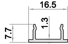
S80-408 AĞIRLIK / WEIGHT (KG/M.) 0,92
