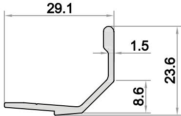
S3-505 AĞIRLIK / WEIGHT (KG/M.) 0,223
