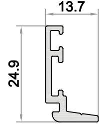
S3-513 AĞIRLIK / WEIGHT (KG/M.) 0,216
