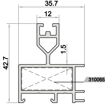
S3-515 AĞIRLIK / WEIGHT (KG/M.) 0,709
