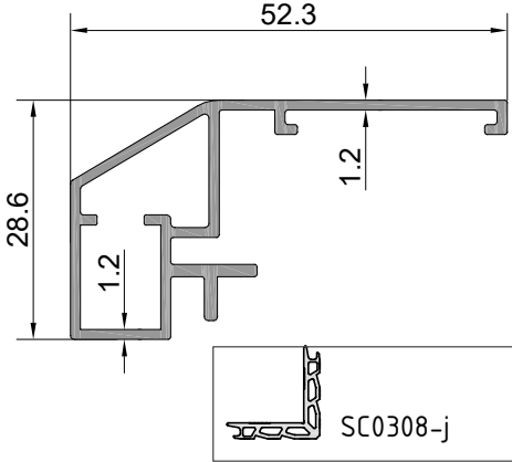
Profil No: OB1-110 Ağırlık : 487 gr/m
